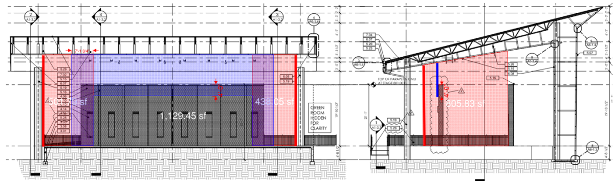
1 STAGE LONGITUDINAL SECTION A1-3.2 SCALE: 1/8" = 1'-0"
