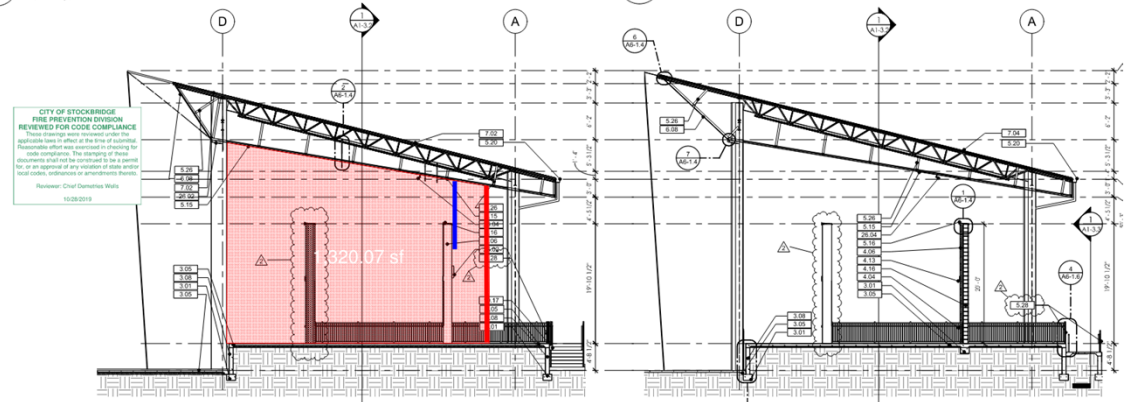
1 STAGE LONGITUDINAL SECTION A1-3.2 SCALE: 1/8" = 1'-0"
